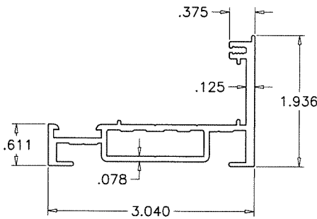
1A FLUSH FRAME HEAD/SILL/JAMB
